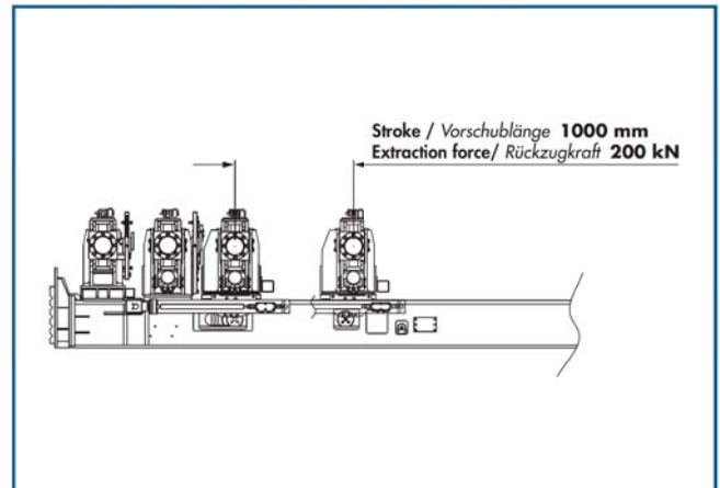
Clamping and breaking devices Klemm- und Brechvorrichtungen
