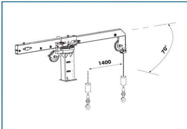
Telescopic and 70° swinging cat head Turmkrone, teleskopierbar und 70° schwenkbar
