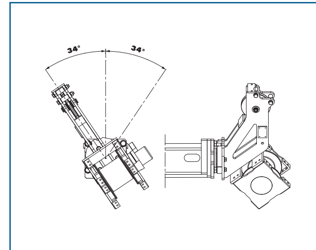
Cat head with winch Turmkrone mit Winde
