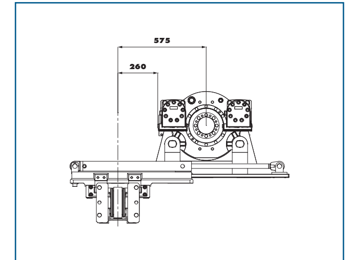
Lateral slide Gleitschlitten seitlich verschiebbar
